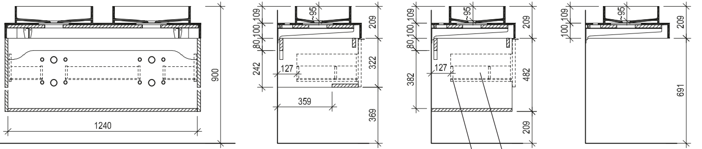
Maßskizze 20
