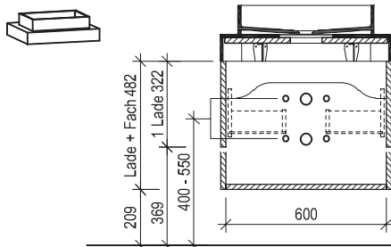
Maßskizze 5
