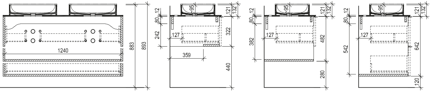
Maßskizze 20
