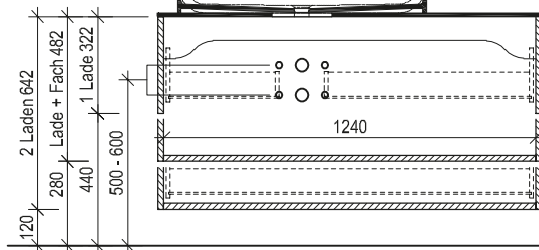
Maßskizze 17
