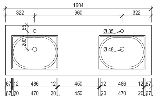
Maßskizze 33
