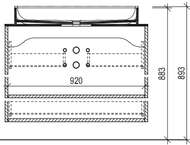
Maßskizze 8
