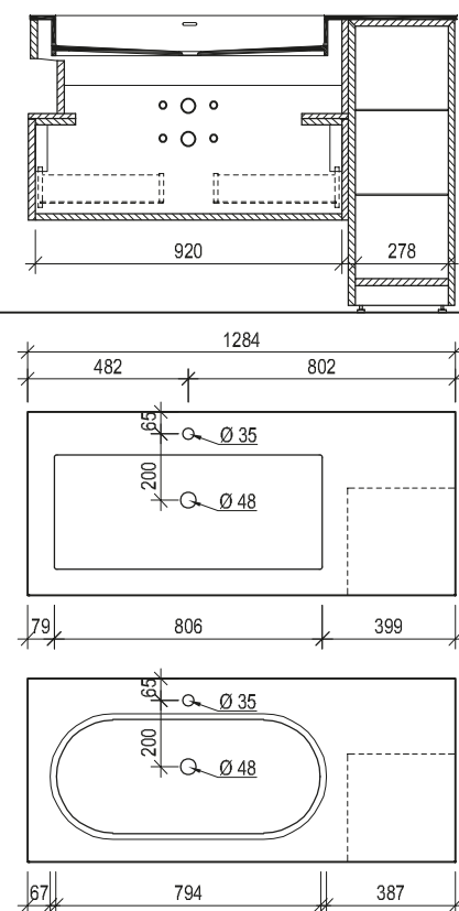
Maßskizze 46
