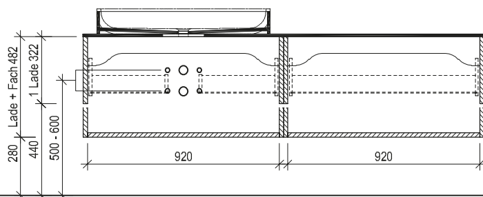
Maßskizze 37
