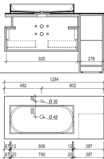
Maßskizze 42
