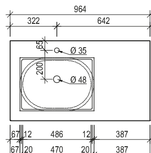
Maßskizze 11
