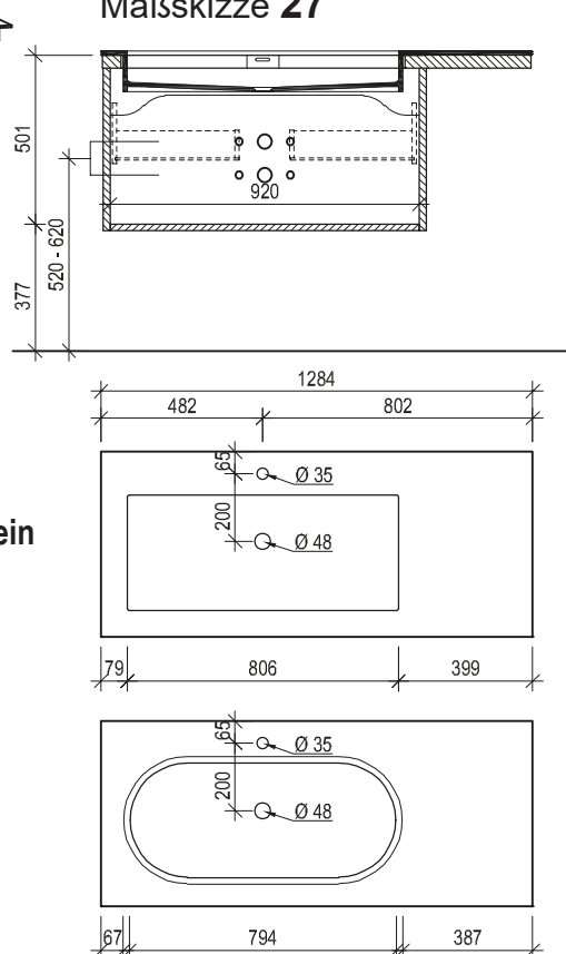
Maßskizze 27
