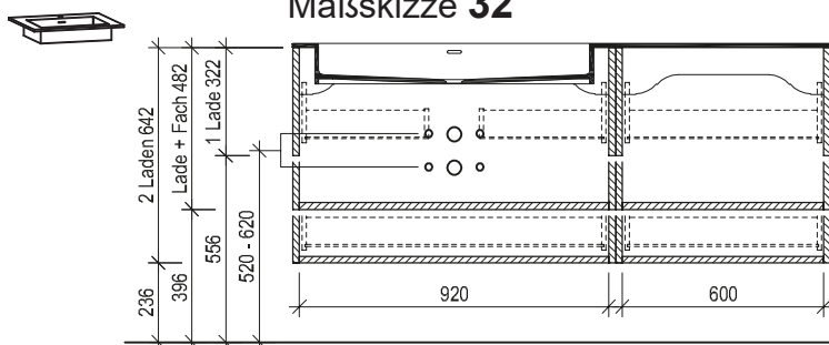
Maßskizze 32
