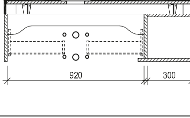
Maßskizze 18
