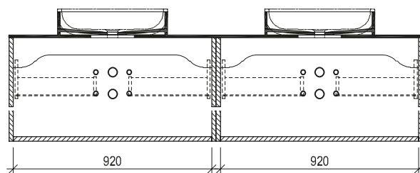
Maßskizze 35
