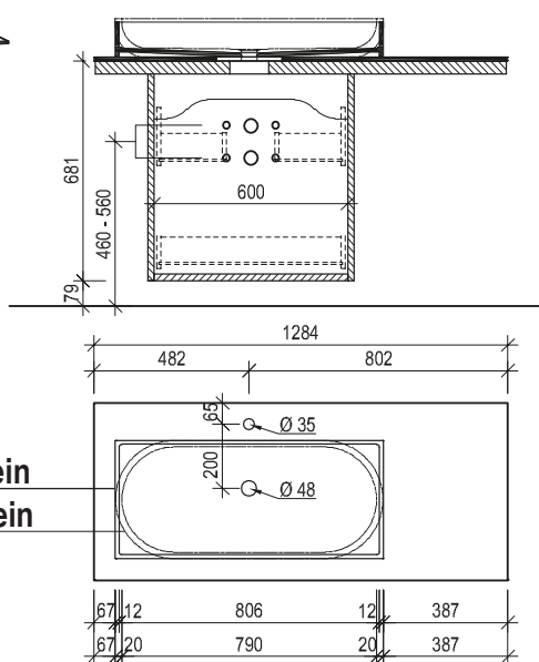
Maßskizze 25
