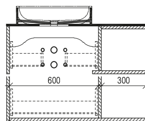
Maßskizze 3
