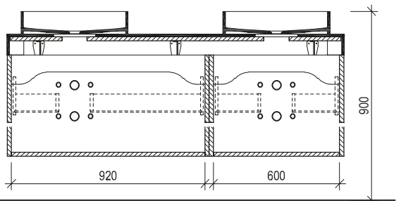
Maßskizze 31
