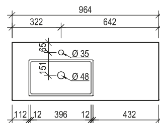
Maßskizze 61
