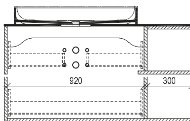
Maßskizze 14
