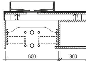
Maßskizze 7
