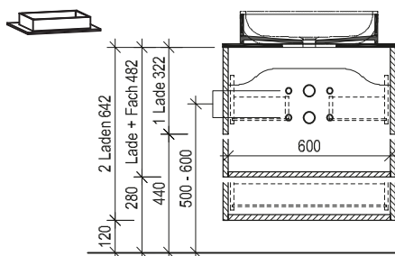
Maßskizze 5
