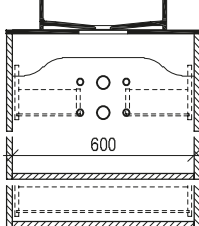
Maßskizze 54
