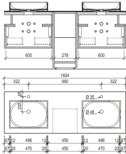
Maßskizze 44
