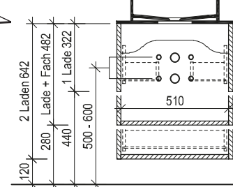
Maßskizze 53
