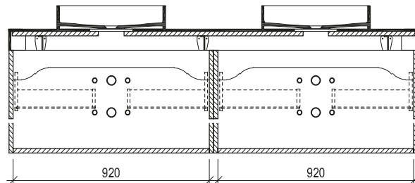
Maßskizze 38
