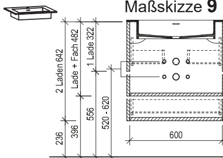
Maßskizze 9
