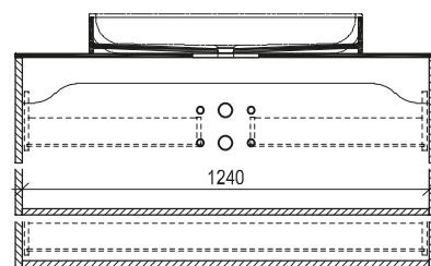
Maßskizze 15
