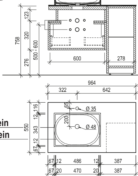
Maßskizze 41
