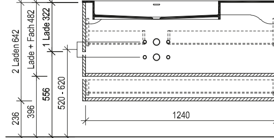
Maßskizze 21
