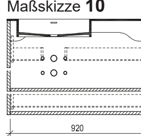
Maßskizze 10
