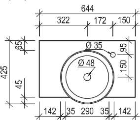
Maßskizze 53
