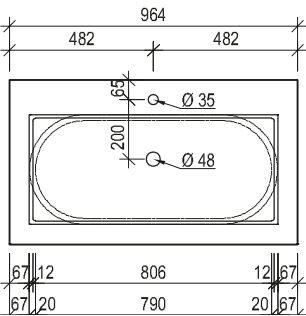
Maßskizze 12
