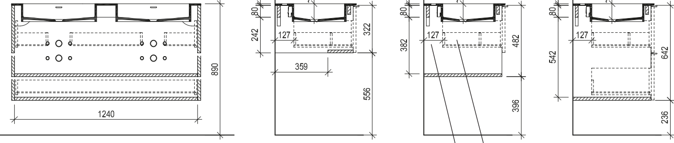
Maßskizze 24
