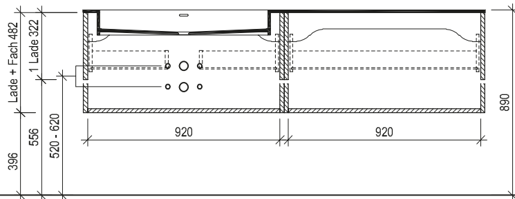
Maßskizze 40
