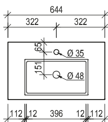
Maßskizze 59
