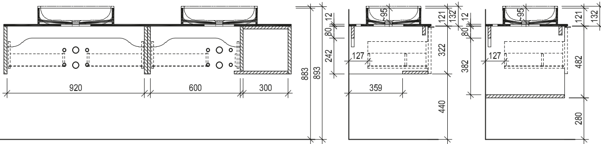
Maßskizze 39
