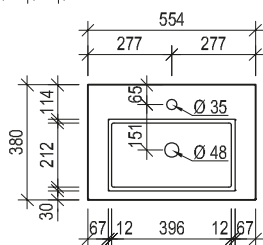
Maßskizze 58
