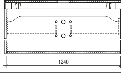
Maßskizze 19
