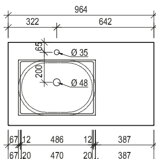
Maßskizze 10
