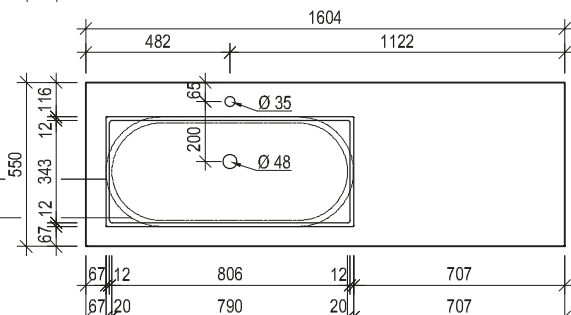
Maßskizze 32
