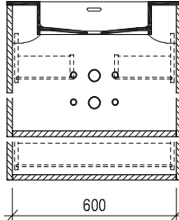
Maßskizze 59
