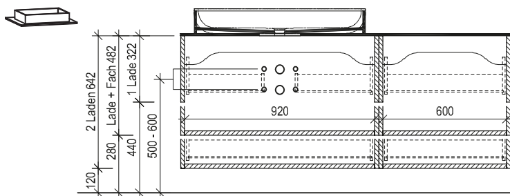
Maßskizze 30
