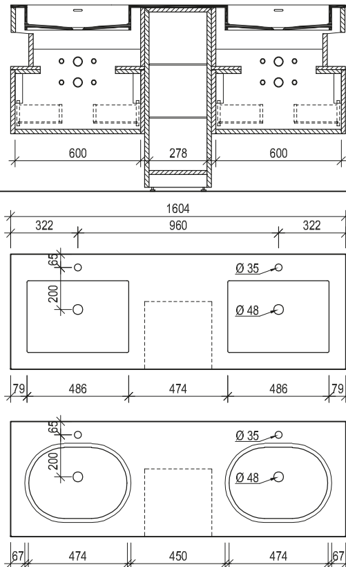
Maßskizze 48
