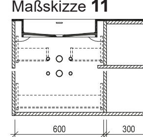
Maßskizze 11
