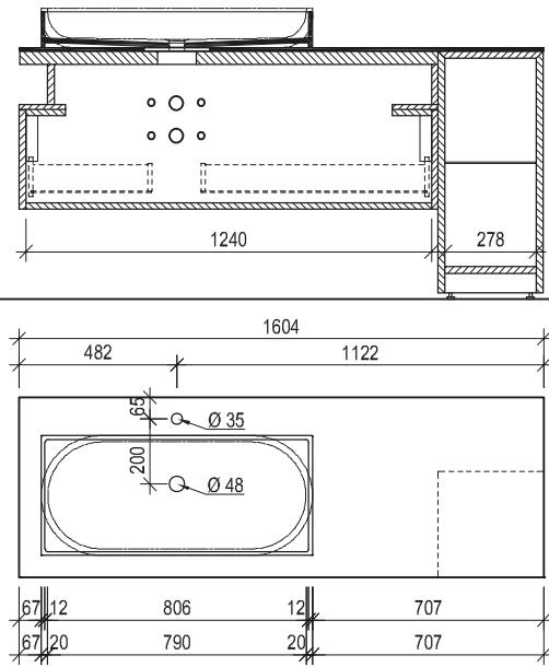
Maßskizze 43
