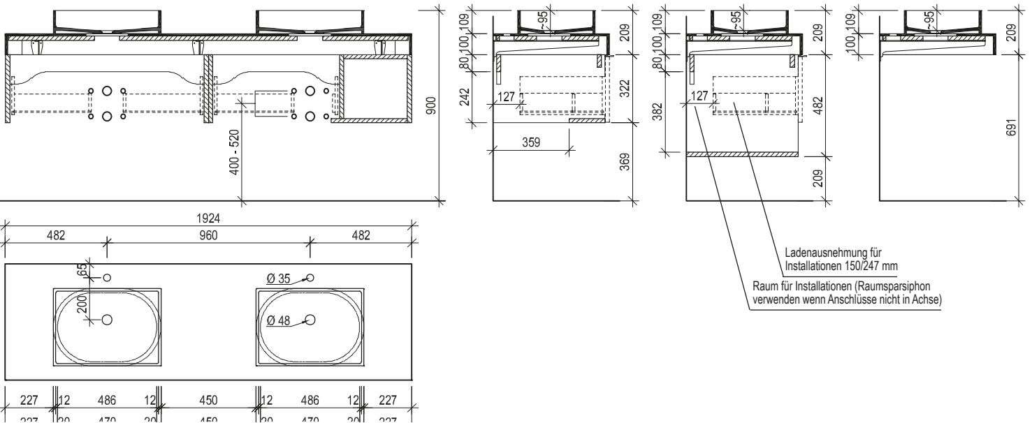
Maßskizze 39
