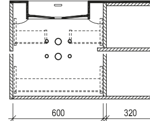
Maßskizze 61
