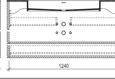
Maßskizze 23
