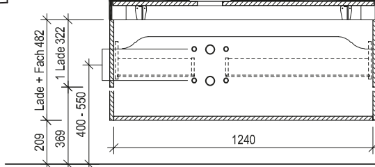
Maßskizze 17
