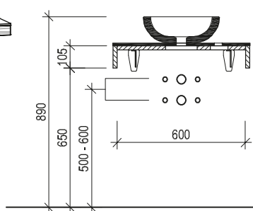
Maßskizze 51
