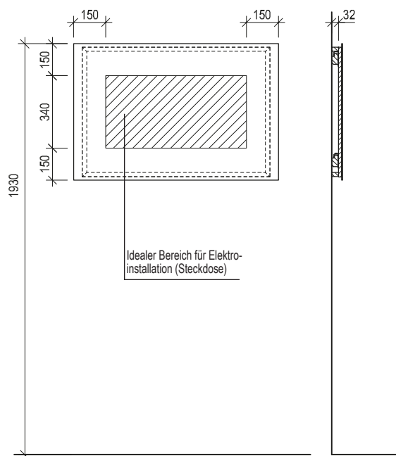
Maßskizze 71
