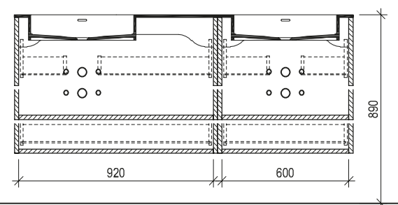
Maßskizze 33
