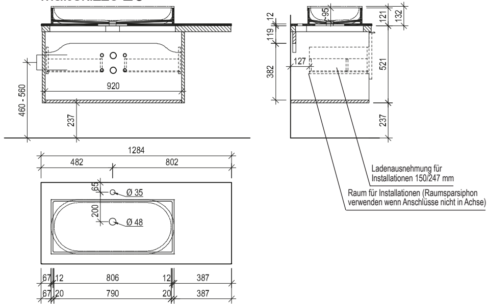
Maßskizze 26
