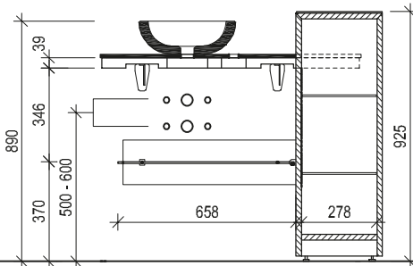
Maßskizze 52
