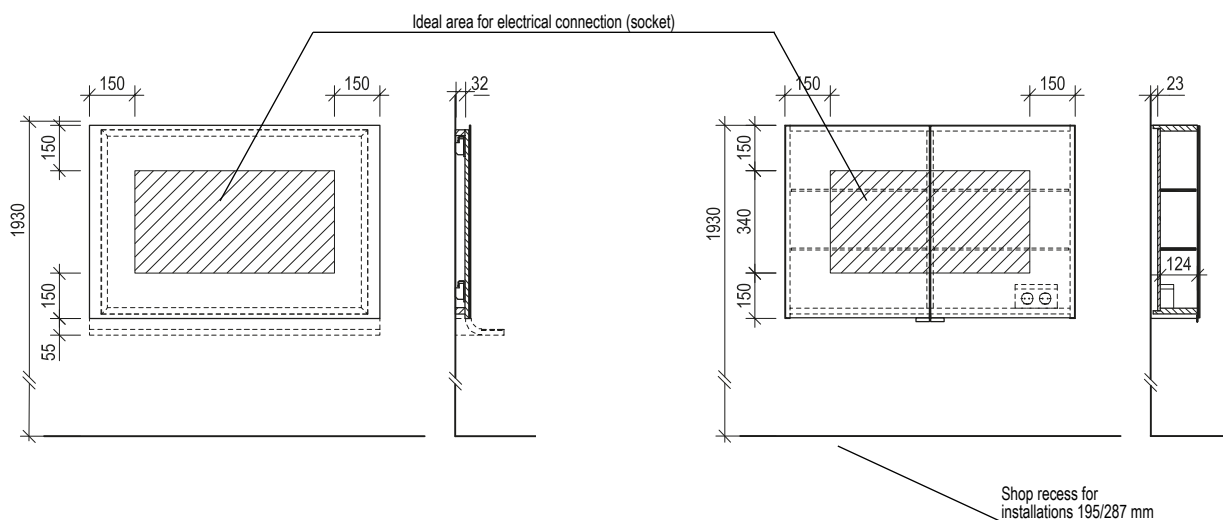
Dim. drawing 12
