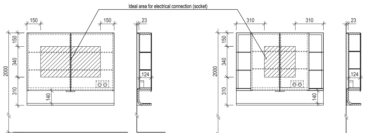
Dim. drawing 14
