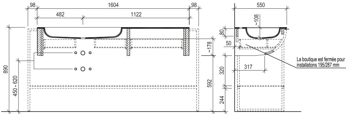
Plan coté 7
