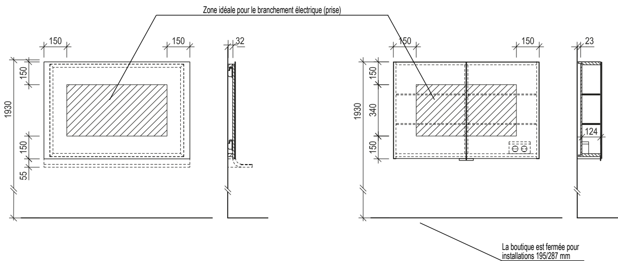
Plan coté 12
