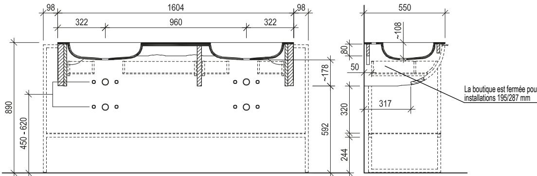
Plan coté 8
