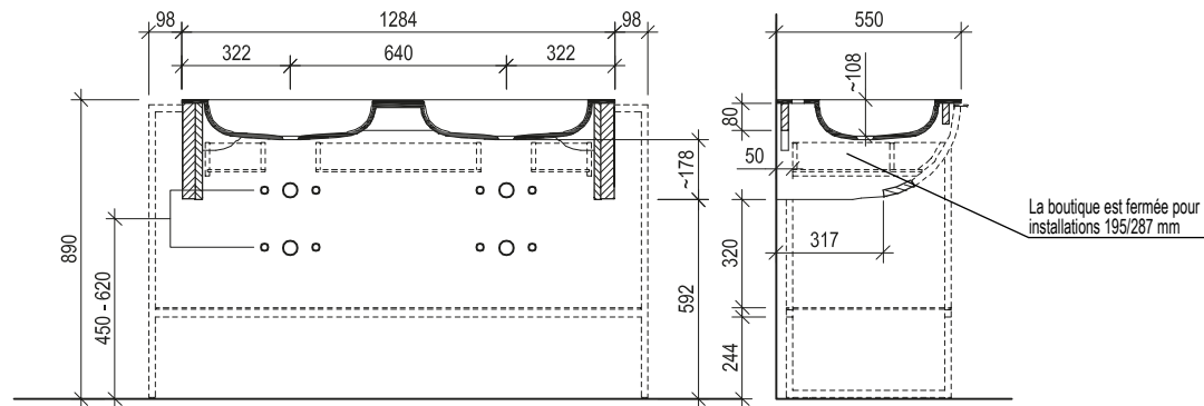
Plan coté 6
