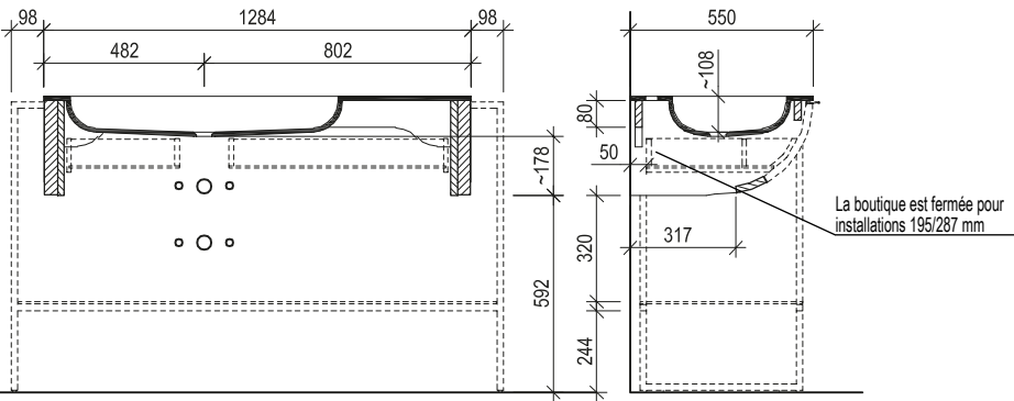
Plan coté 5
