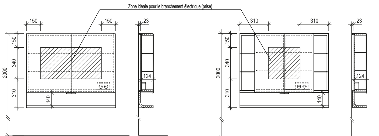
Plan coté 14
