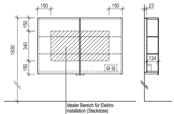
Maßskizze 25
