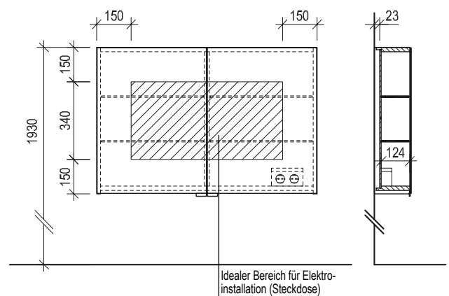
Maßskizze 27
