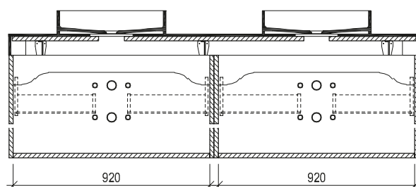
Maßskizze 38
