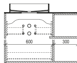
Maßskizze 3
