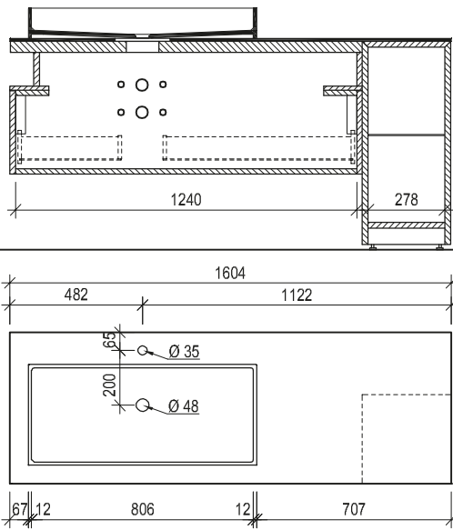
Maßskizze 43
