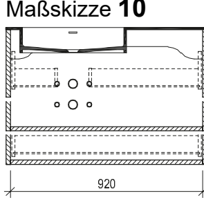
Maßskizze 10
