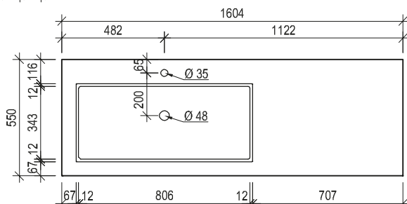
Maßskizze 32
