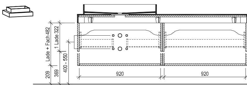
Maßskizze 37
