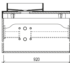
Maßskizze 6
