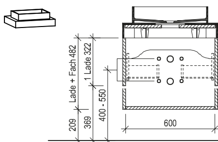
Maßskizze 5
