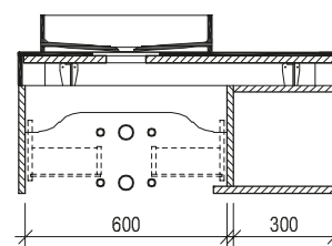
Maßskizze 7
