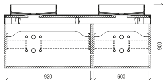
Maßskizze 31
