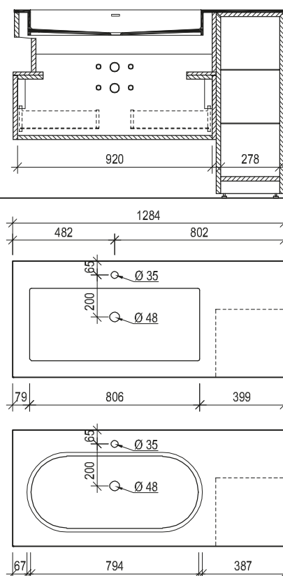
Maßskizze 46
