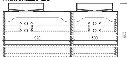
Maßskizze 29
