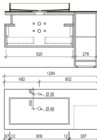
Maßskizze 42
