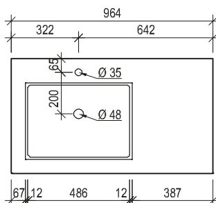
Maßskizze 11
