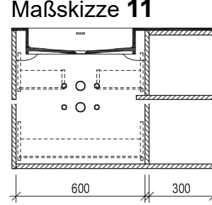
Maßskizze 11
