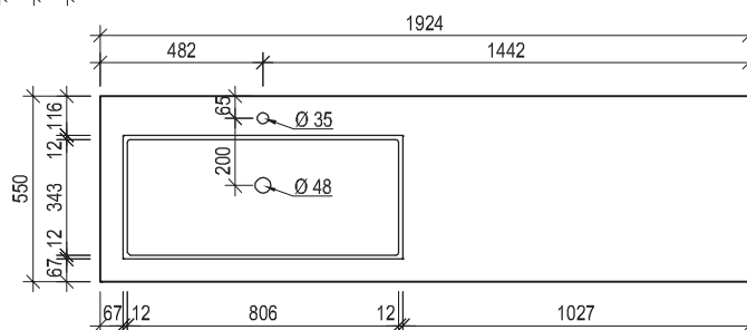
Maßskizze 40
