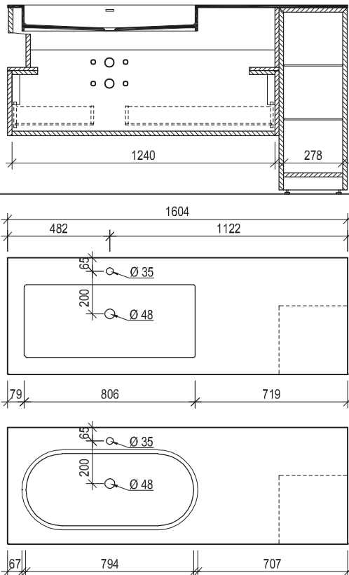
Maßskizze 47
