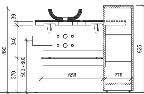
Maßskizze 52
