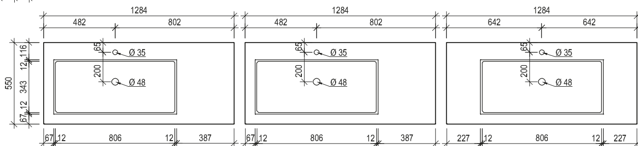
Maßskizze 21
