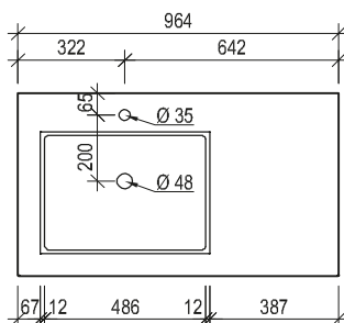
Maßskizze 10
