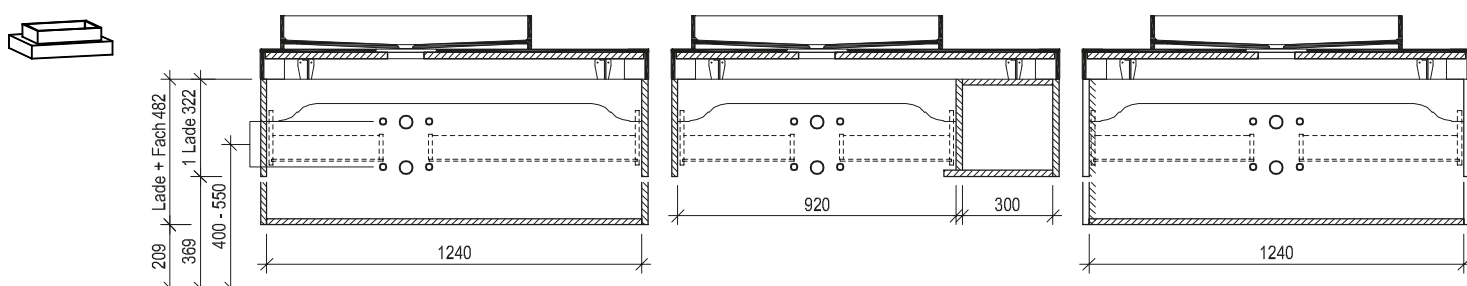
Maßskizze 17
