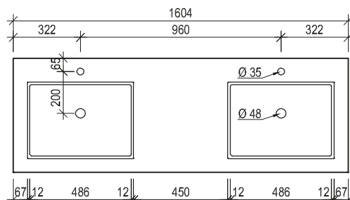
Maßskizze 33
