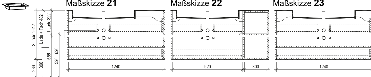
Maßskizze 21
