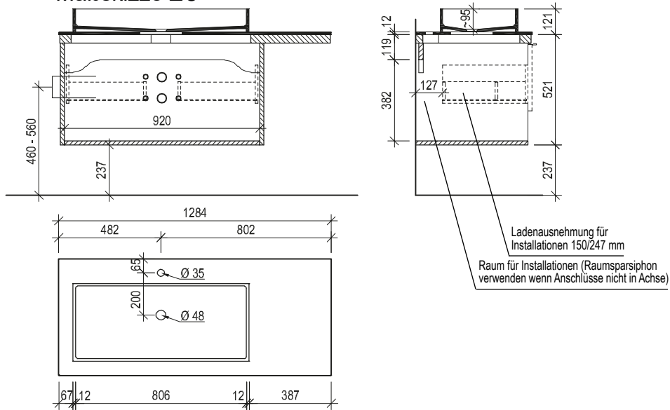
Maßskizze 26
