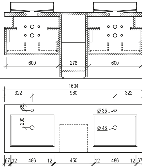
Maßskizze 44
