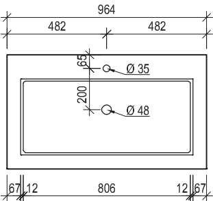
Maßskizze 12
