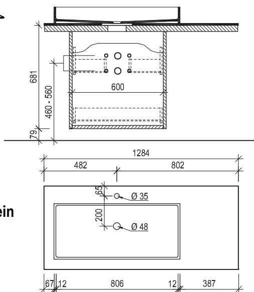
Maßskizze 25
