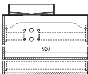
Maßskizze 2
