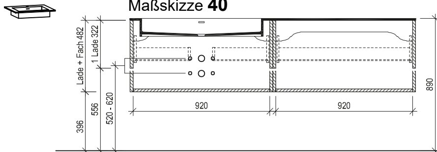
Maßskizze 40
