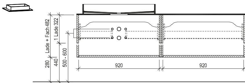
Maßskizze 37
