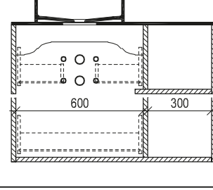
Maßskizze 56
