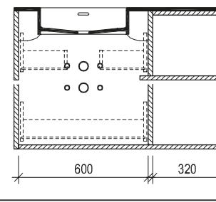
Maßskizze 61
