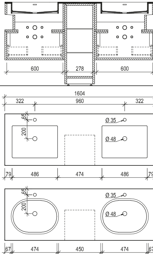
Maßskizze 48
