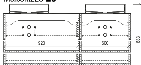
Maßskizze 29
