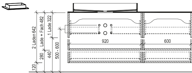
Maßskizze 30
