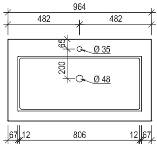
Maßskizze 12
