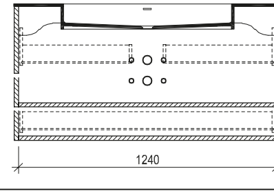
Maßskizze 23
