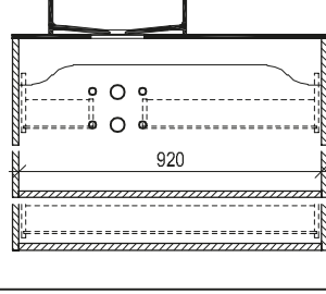
Maßskizze 55
