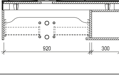
Maßskizze 18
