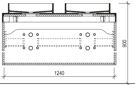
Maßskizze 20
