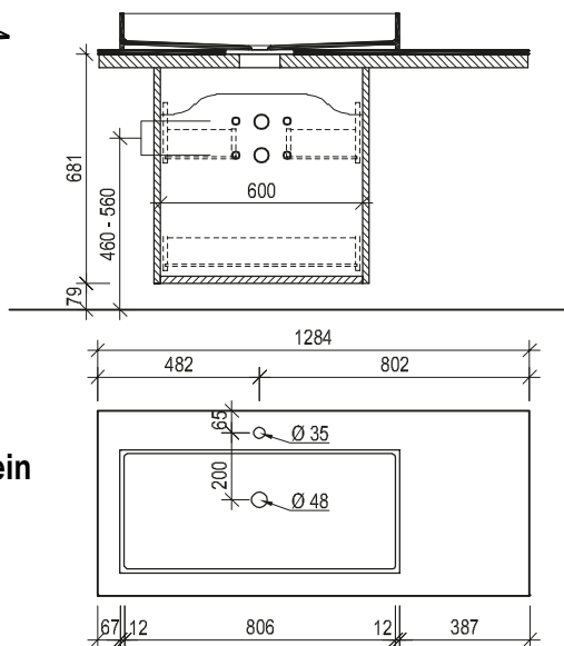
Maßskizze 25
