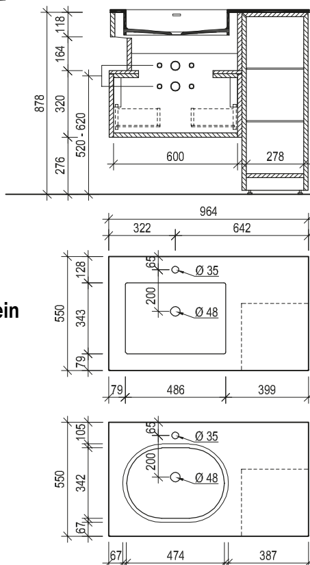
Maßskizze 45
