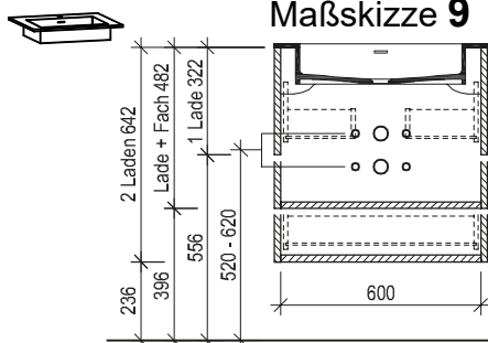
Maßskizze 9
