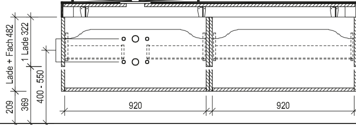
Maßskizze 37
