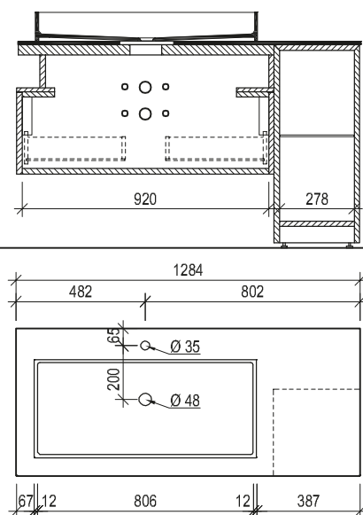
Maßskizze 42
