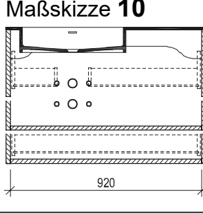
Maßskizze 10
