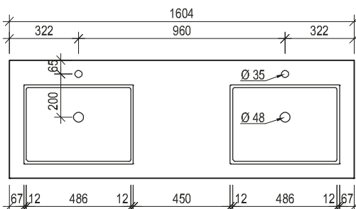
Maßskizze 33
