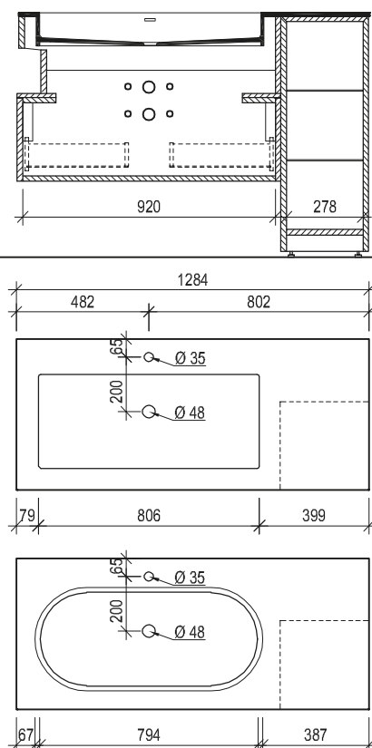
Maßskizze 46
