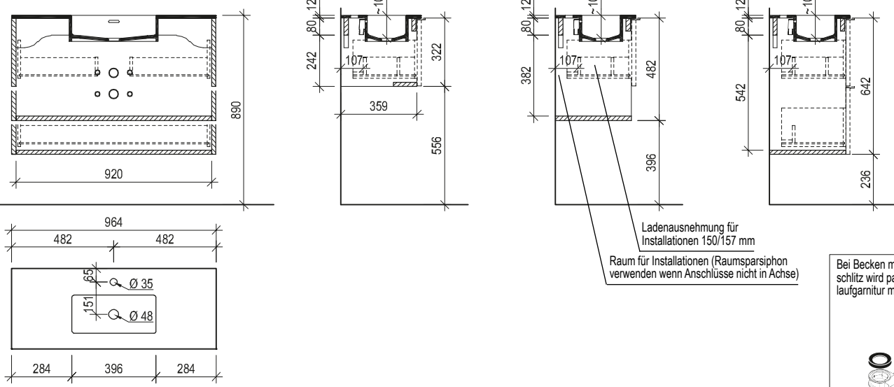
Maßskizze 62
