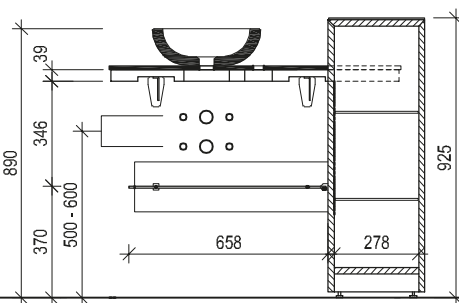
Maßskizze 52
