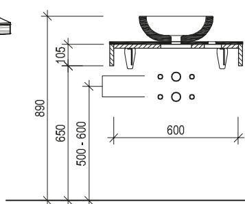
Maßskizze 51
