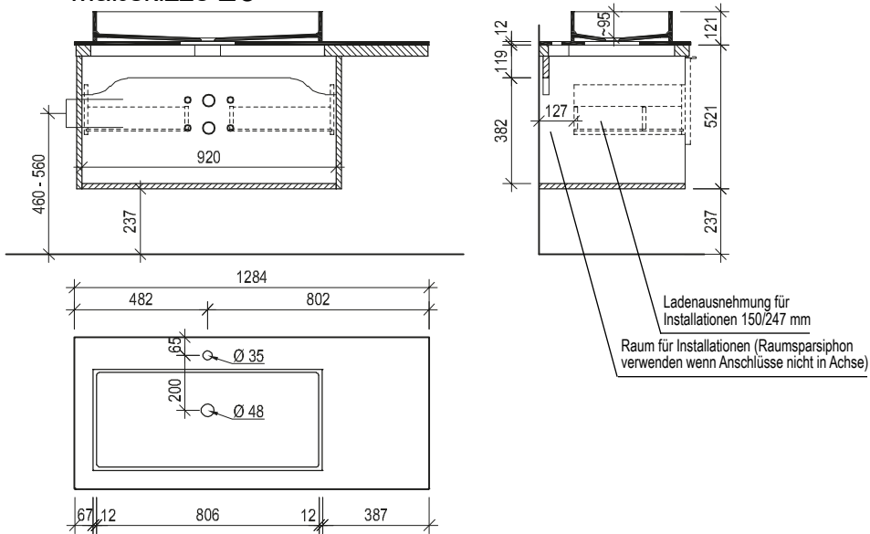
Maßskizze 26
