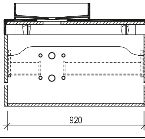
Maßskizze 6
