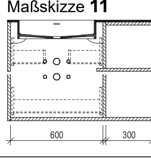
Maßskizze 11
