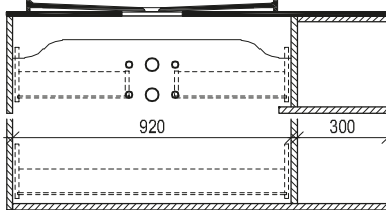
Maßskizze 18
