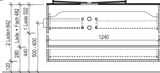
Maßskizze 17
