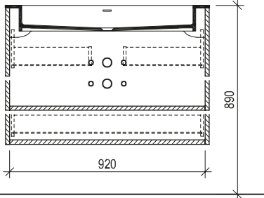
Maßskizze 12
