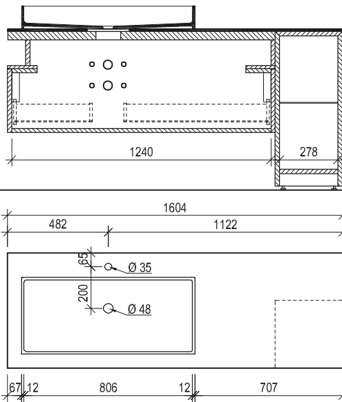
Maßskizze 43
