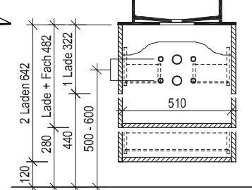
Maßskizze 53
