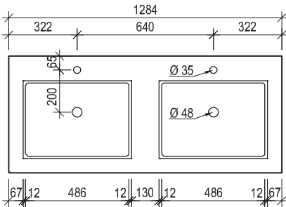
Maßskizze 24
