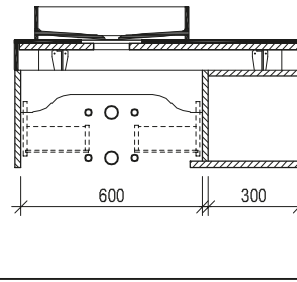
Maßskizze 7
