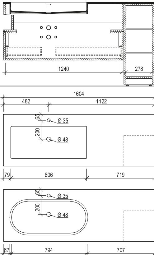
Maßskizze 47
