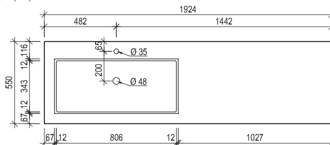
Maßskizze 40
