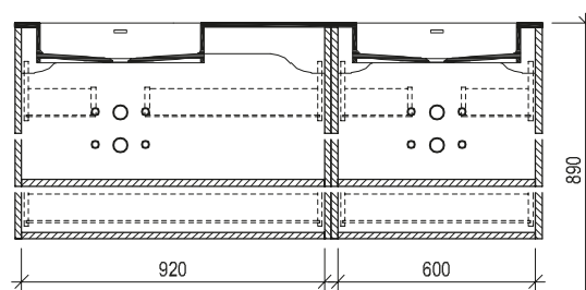
Maßskizze 33
