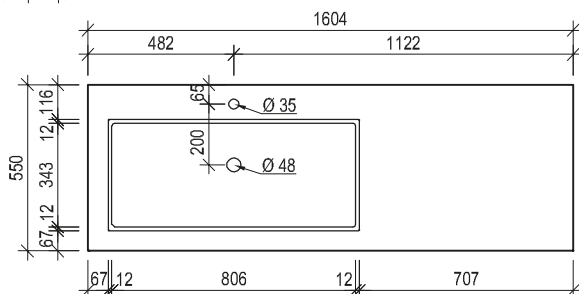
Maßskizze 32
