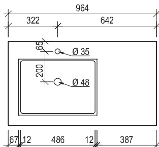
Maßskizze 10
