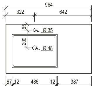
Maßskizze 11
