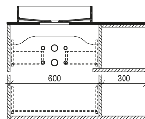
Maßskizze 3
