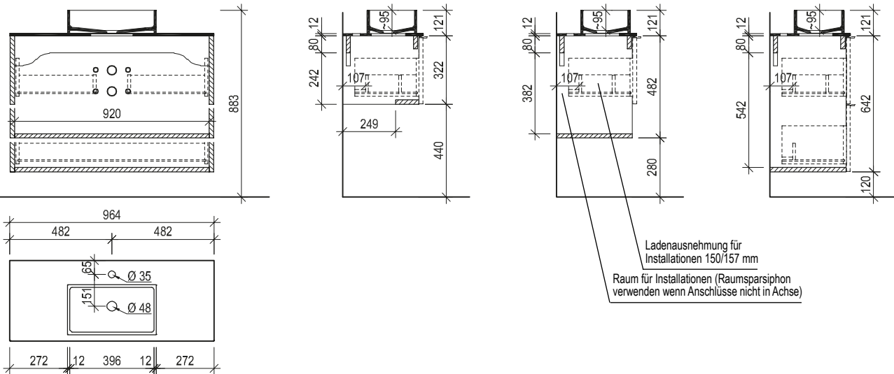
Maßskizze 57
