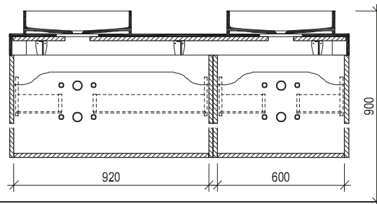
Maßskizze 31
