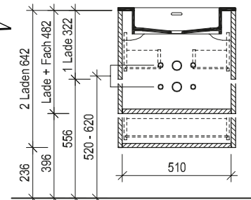
Maßskizze 58
