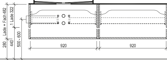
Maßskizze 37
