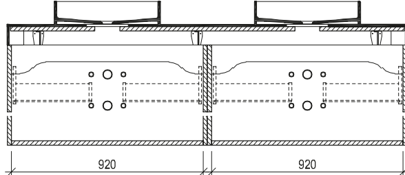
Maßskizze 38
