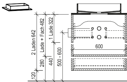
Maßskizze 5
