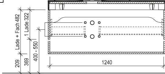
Maßskizze 17
