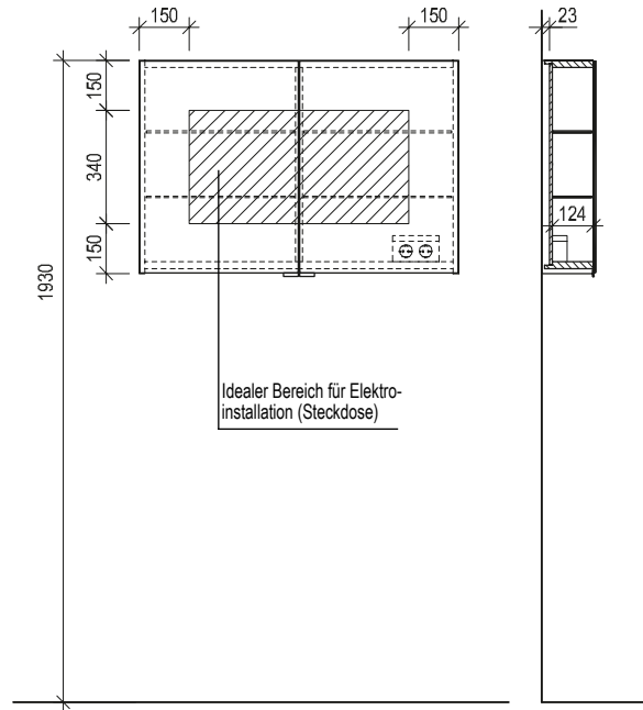
Maßskizze 72
