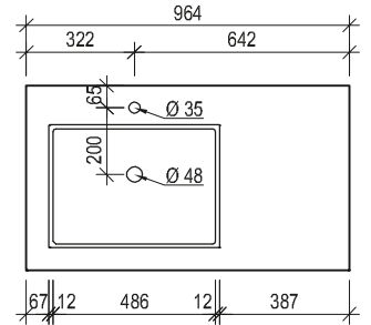
Maßskizze 11
