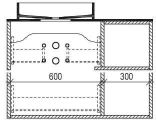
Maßskizze 3
