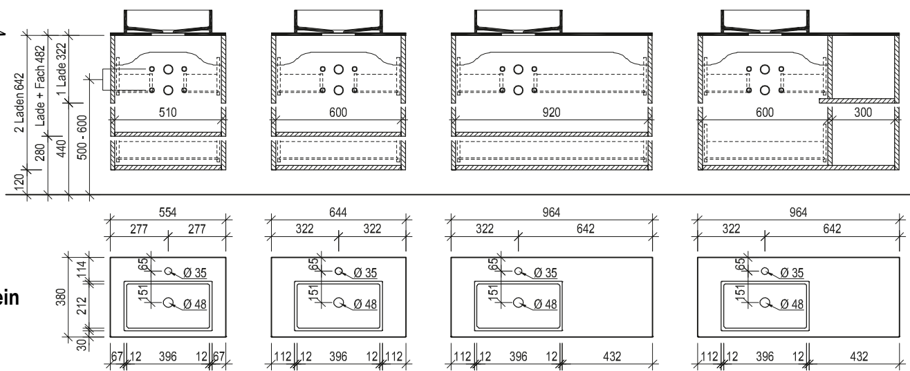
Maßskizze 54
