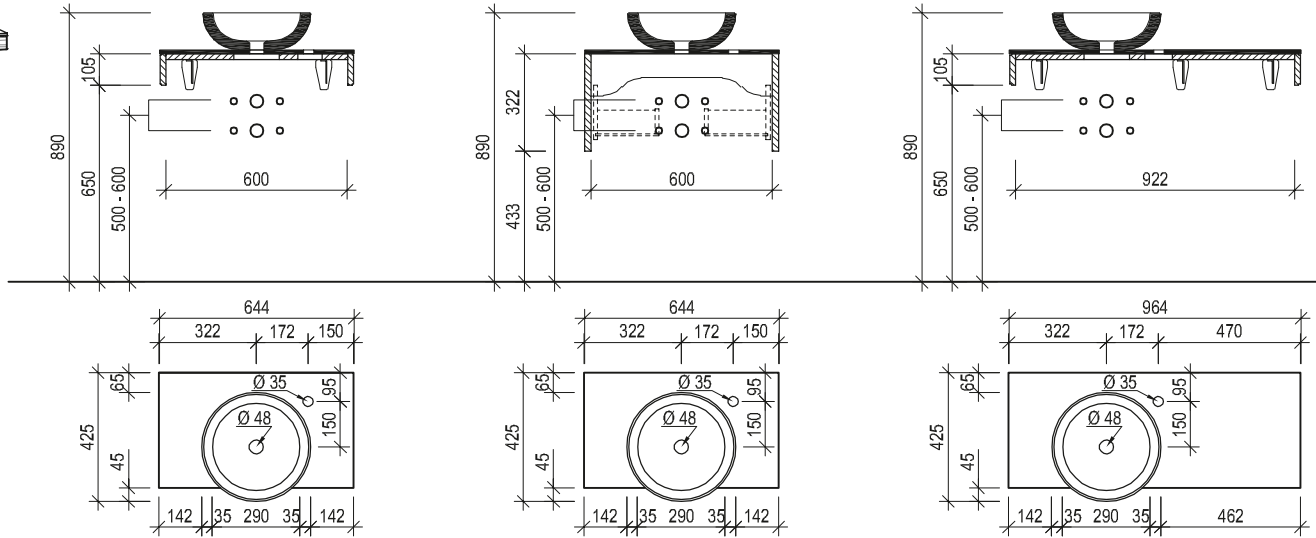
Maßskizze 51
