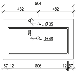
Maßskizze 12
