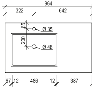
Maßskizze 10
