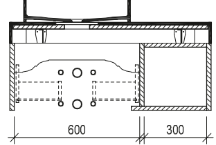
Maßskizze 7
