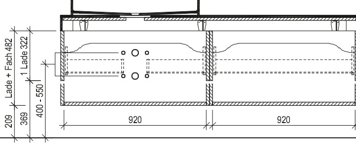
Maßskizze 34
