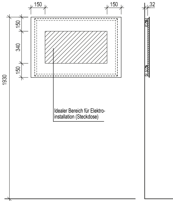
Maßskizze 71
