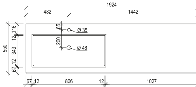
Maßskizze 37
