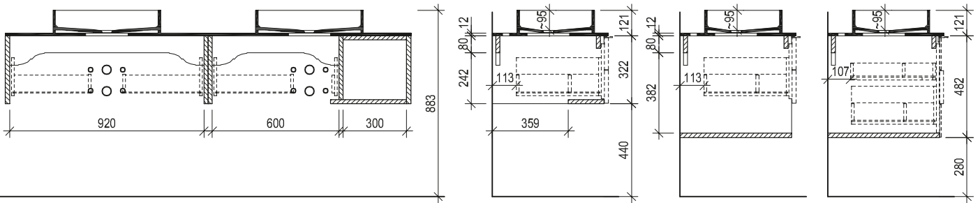
Maßskizze 36
