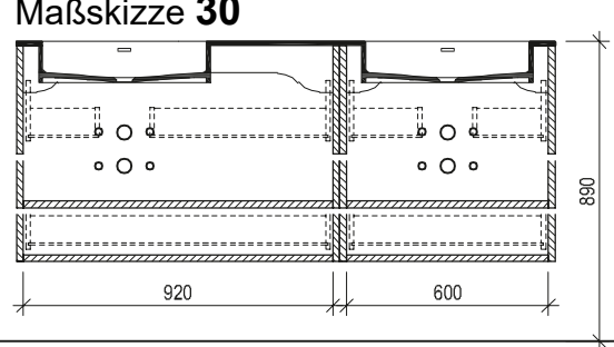
Maßskizze 30
