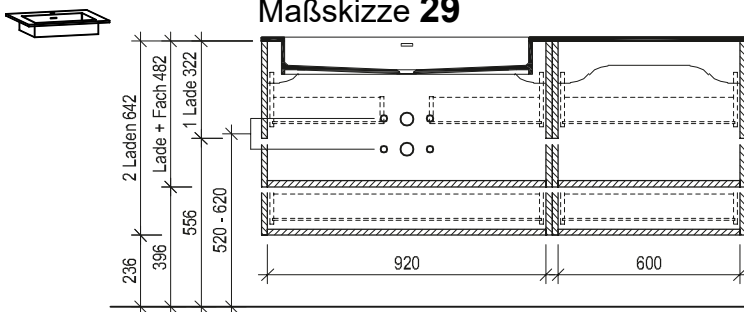
Maßskizze 29
