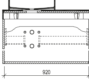
Maßskizze 6
