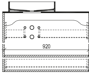
Maßskizze 2
