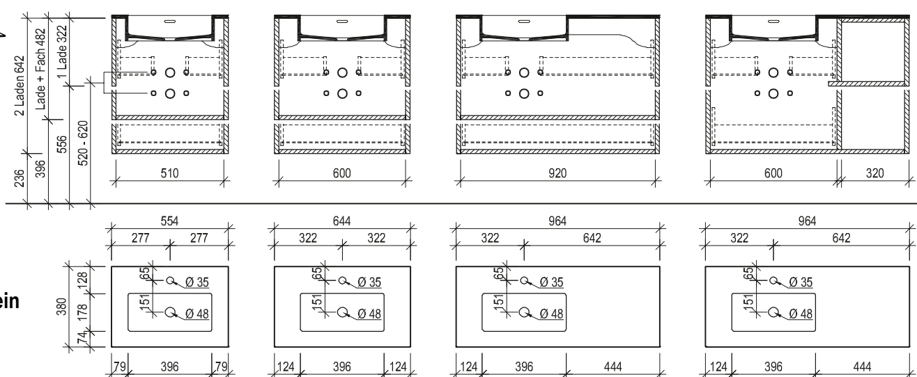
Maßskizze 59
