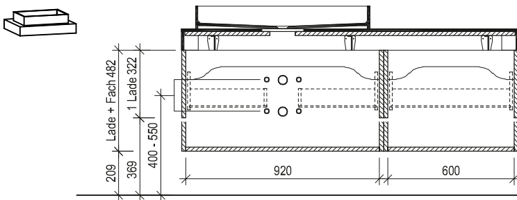
Maßskizze 27
