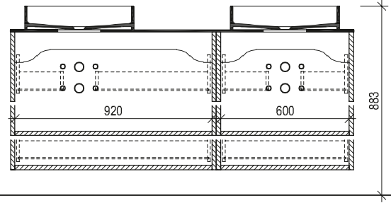
Maßskizze 28
