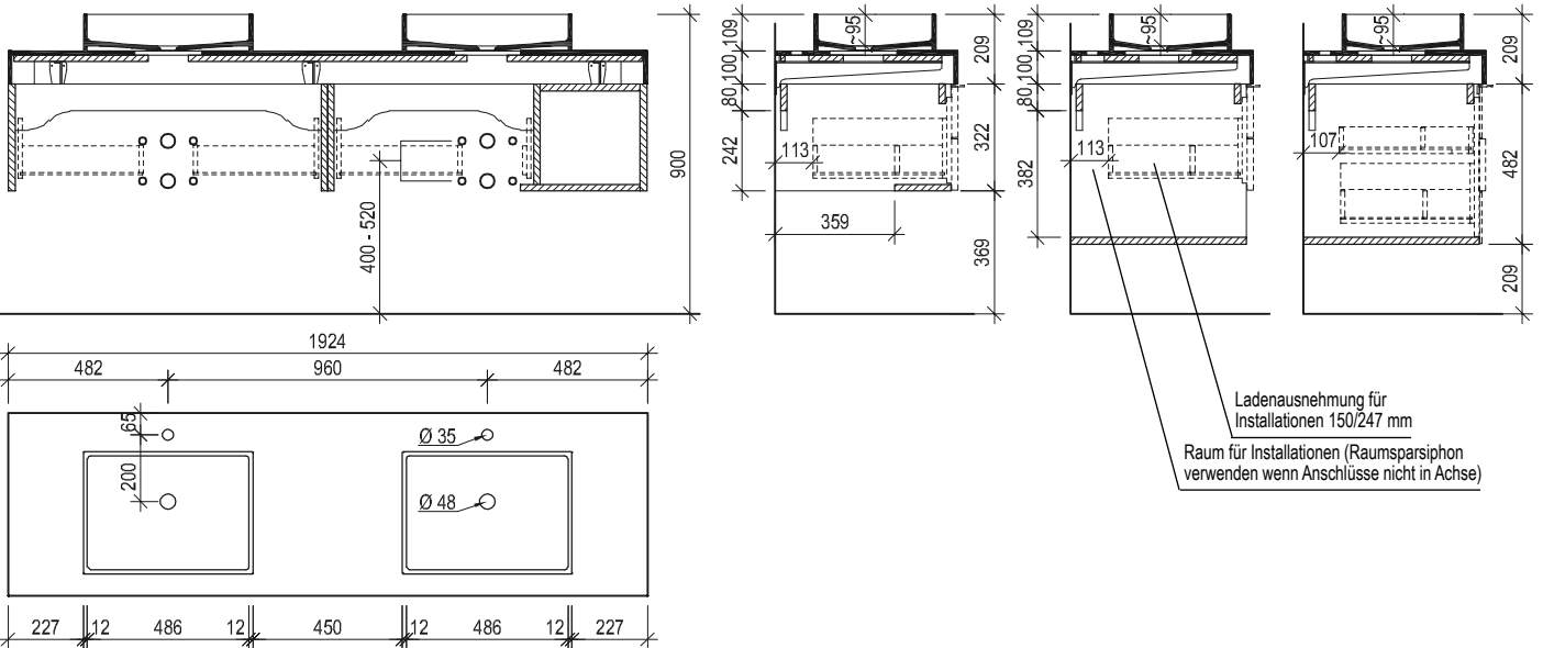
Maßskizze 36
