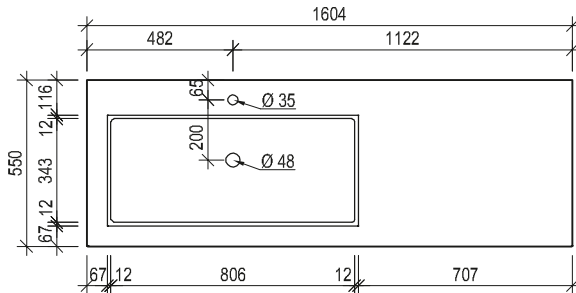
Maßskizze 29
