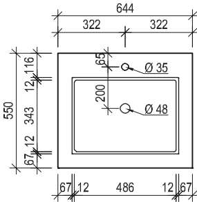
Maßskizze 9
