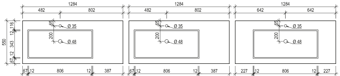
Maßskizze 21
