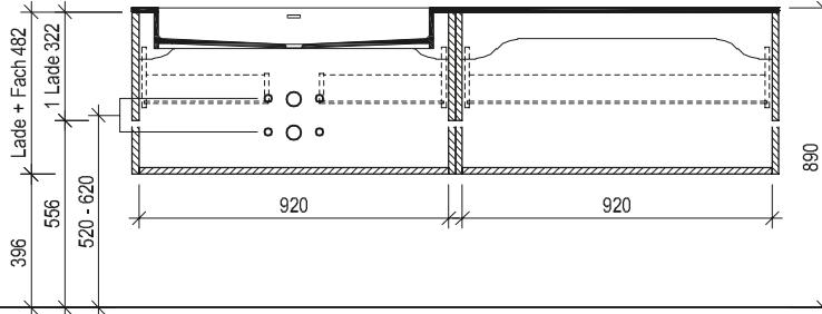
Maßskizze 37
