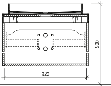
Maßskizze 8
