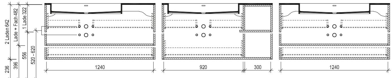
Maßskizze 21
