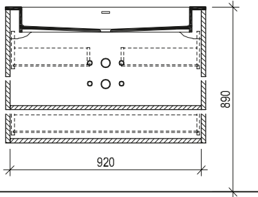
Maßskizze 12
