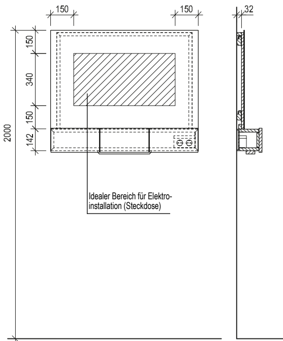
Maßskizze 73
