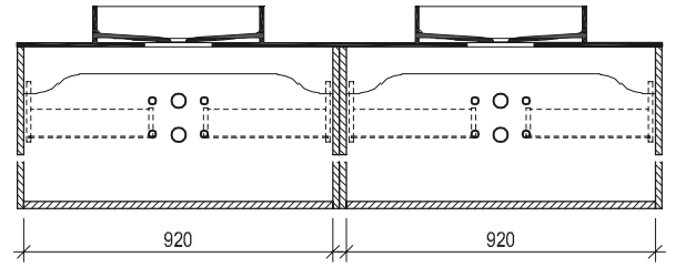
Maßskizze 32
