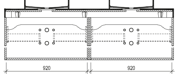
Maßskizze 35
