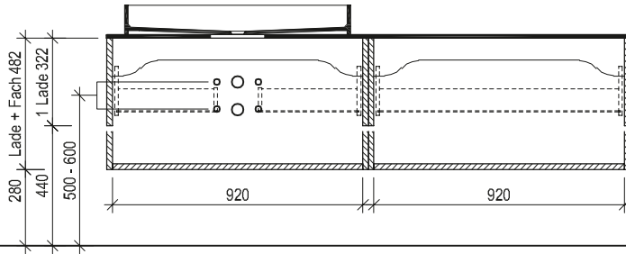
Maßskizze 34
