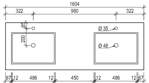
Maßskizze 30
