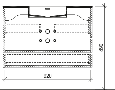
Maßskizze 63
