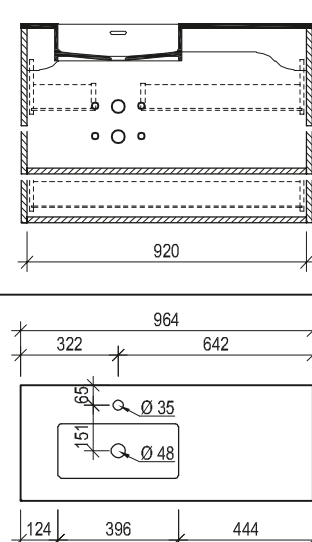
Maßskizze 61
