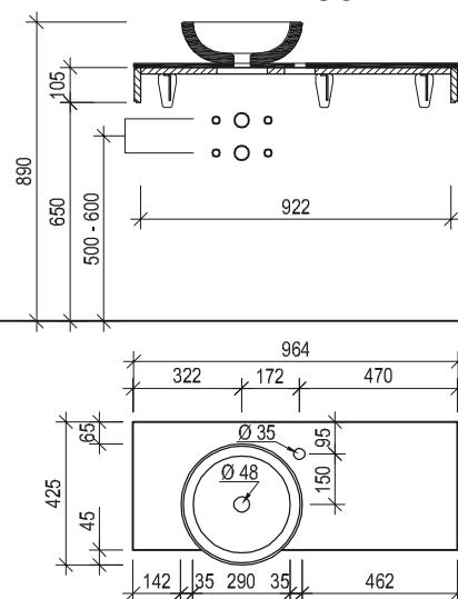
Maßskizze 53
