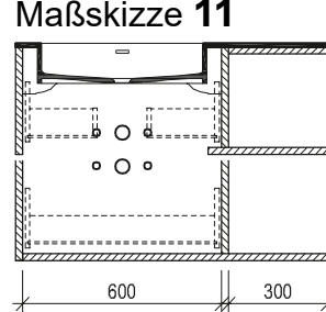
Maßskizze 11
