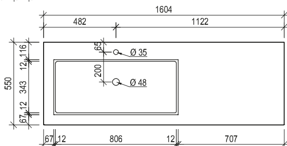
Maßskizze 29
