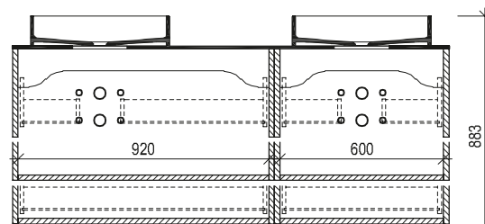
Maßskizze 26
