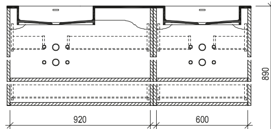
Maßskizze 30
