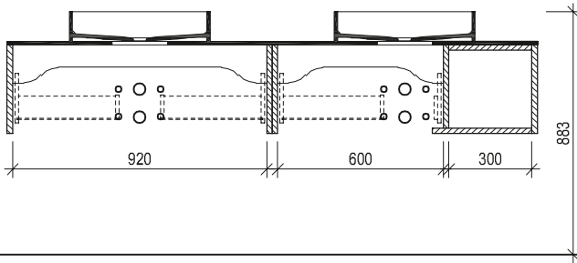
Maßskizze 36
