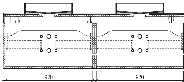
Maßskizze 35
