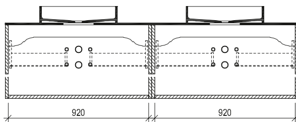
Maßskizze 32
