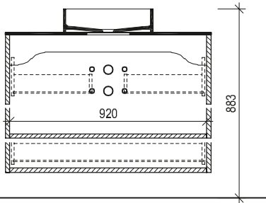
Maßskizze 58
