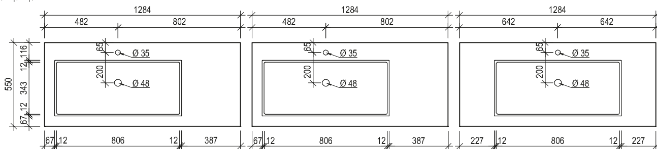
Maßskizze 21
