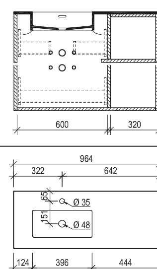
Maßskizze 62
