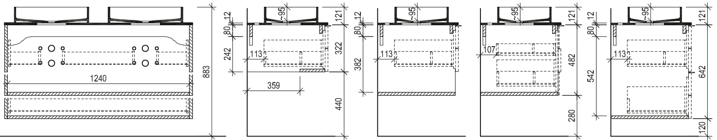
Maßskizze 20
