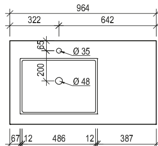
Maßskizze 11
