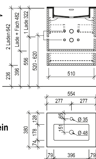
Maßskizze 59
