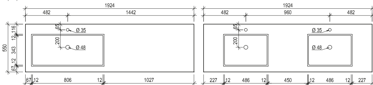
Maßskizze 37
