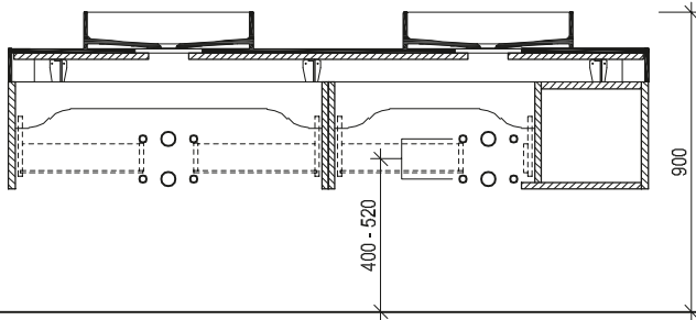
Maßskizze 36
