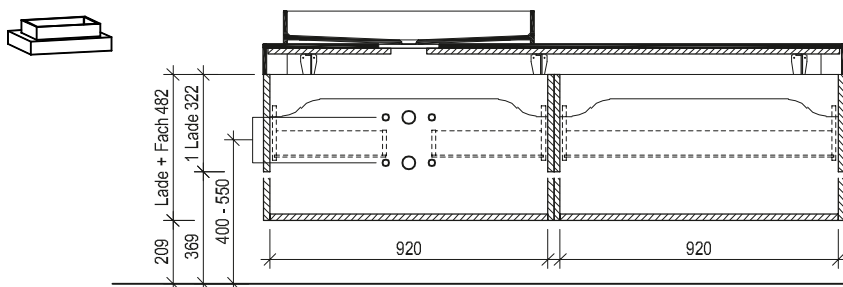
Maßskizze 34
