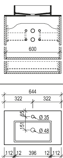
Maßskizze 55
