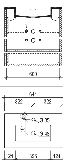
Maßskizze 60
