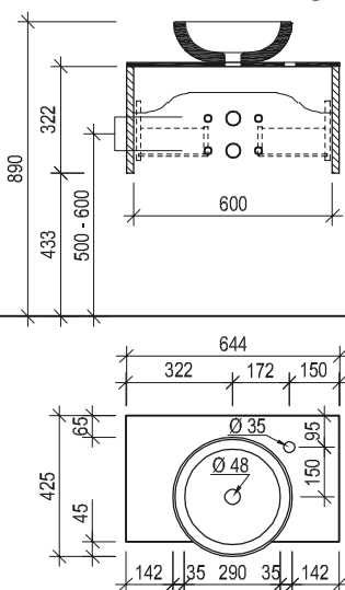
Maßskizze 52
