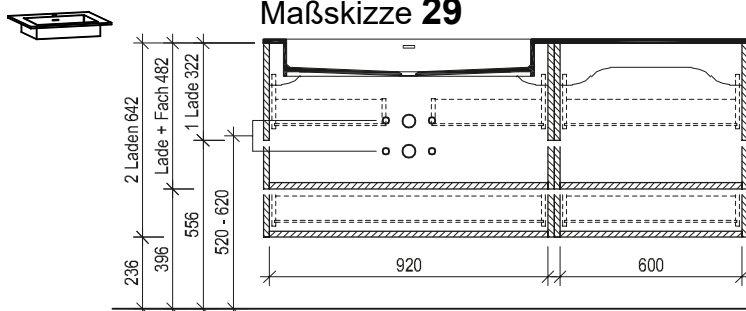
Maßskizze 29
