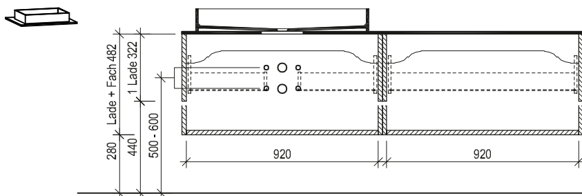
Maßskizze 34
