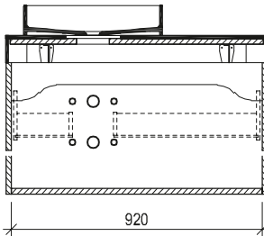
Maßskizze 6
