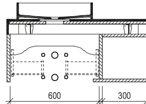
Maßskizze 7
