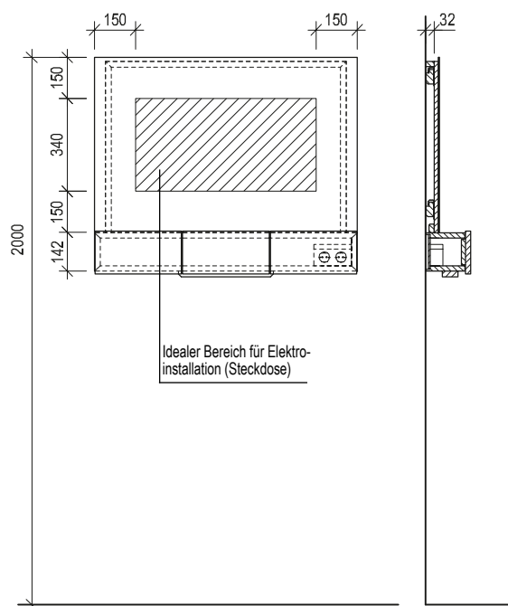
Maßskizze 73
