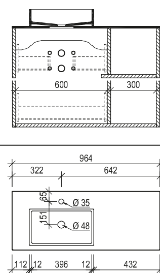
Maßskizze 57
