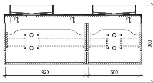
Maßskizze 28
