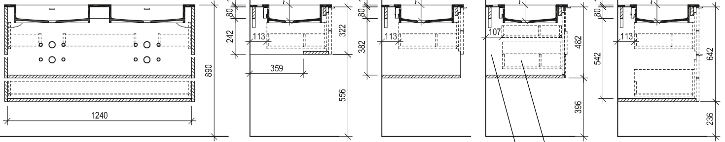
Maßskizze 24
