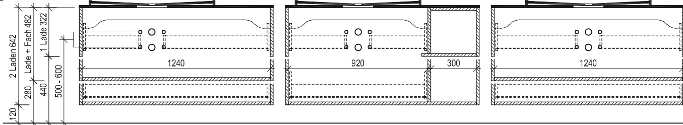
Maßskizze 17
