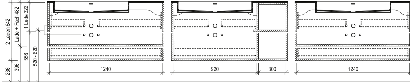
Maßskizze 21
