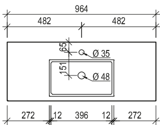
Maßskizze 63
