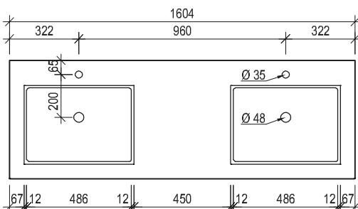
Maßskizze 30
