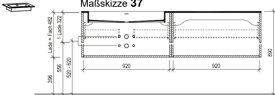
Maßskizze 37
