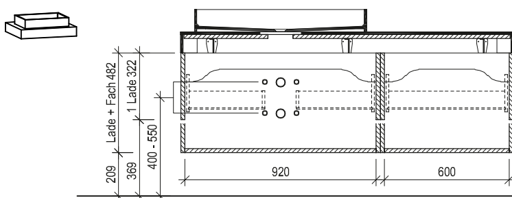
Maßskizze 27
