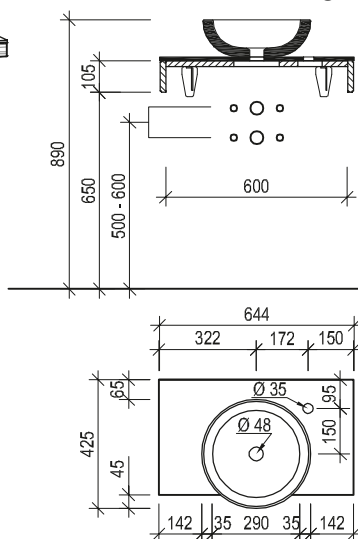
Maßskizze 51
