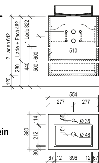
Maßskizze 54
