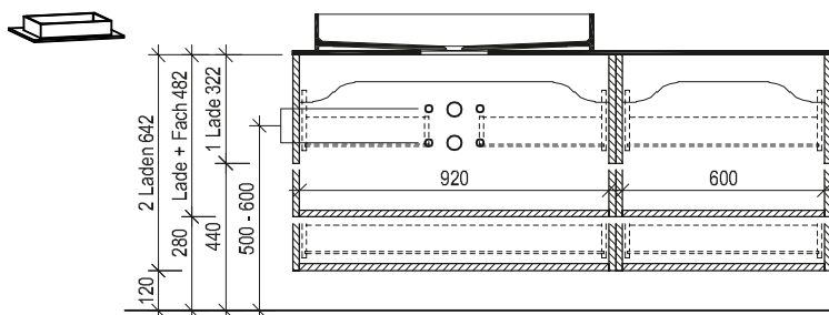
Maßskizze 27
