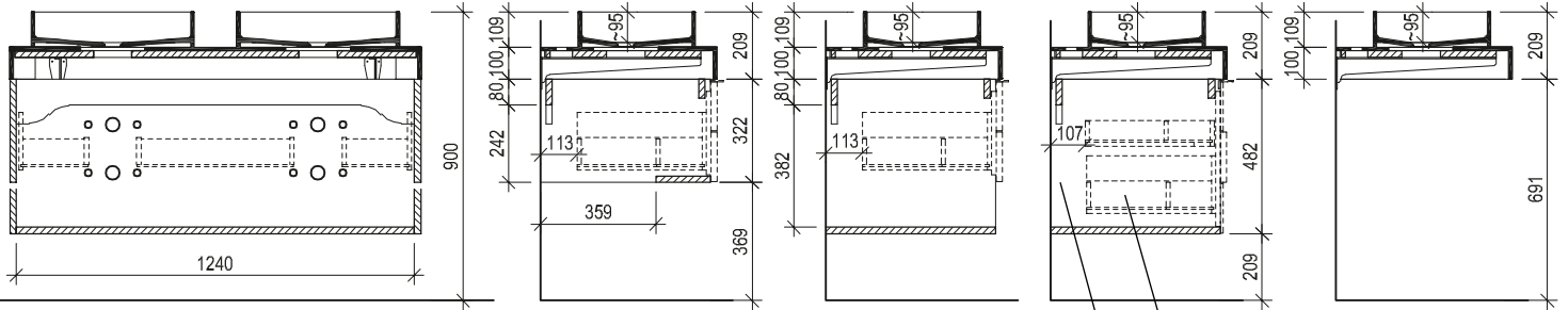
Maßskizze 20
