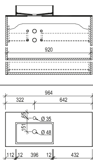
Maßskizze 56
