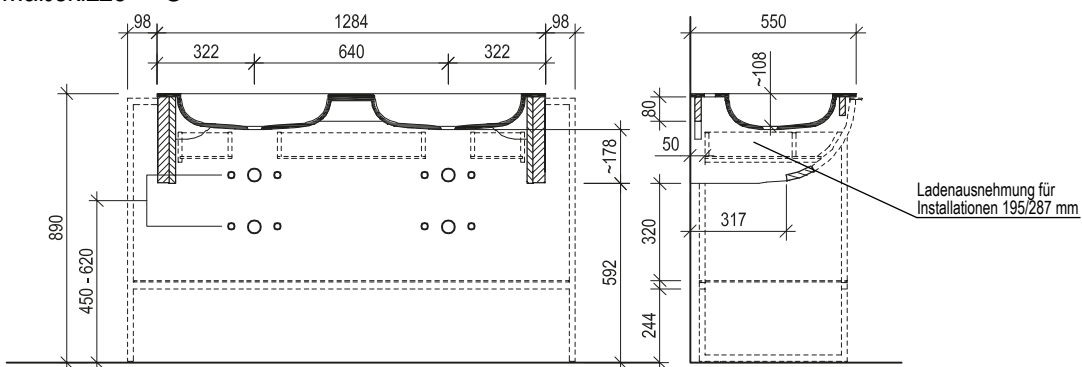
Maßskizze 6
