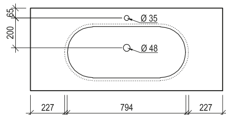
Maßskizze 6
