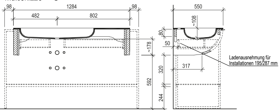
Maßskizze 5
